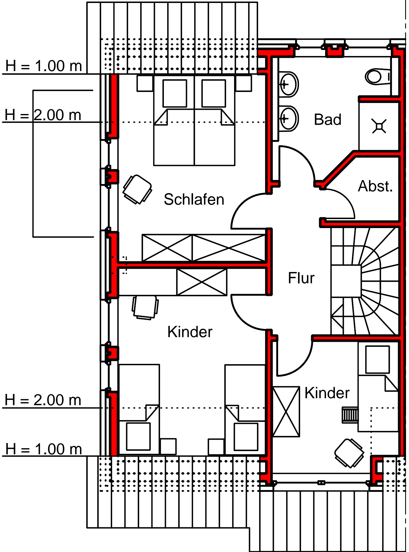
Dachgeschoss
